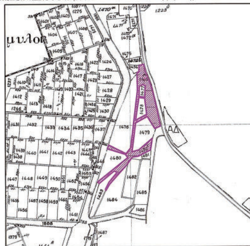
ΑΠΟΣΠΑΣΜΑ ΠΡΟΣΕΓΓΙΣΤΙΚΗΣ ΘΕΣΗΣ ΚΕΝΤΡΙΚΟΥ ΑΝΤΛΙΩΣΤΑΣΙΟΥ ΠΥΡΟΣΒΕΣΗΣ ΣΕ ΥΠΟΒΑΘΡΟ ΣΥΜΠΛΗΡΩΜΑΤΙΚΗΣ ΔΙΑΝΟΜΗΣ ΚΡΗΝΙΔΩΝ ΕΤΟΥΣ 1957 (ΕΝΤΟΣ ΕΥΡΥΤΕΡΟΥ ΤΕΜΑΧΙΟΥ 1470 στ (πρώην 1470 γ))
