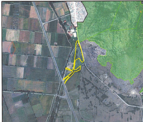
ΑΠΟΣΠΑΣΜΑ ΘΕΣΗΣ ΚΕΝΤΡΙΚΟΥ ΑΝΤΙΔΙΟΤΑΣΙΟΥ ΠΥΡΟΣΒΕΣΗΣ ΣΕ ΟΡΘΟΦΩΤΟΧΑΡΤΗ ΤΗΣ ΕΚΔΑ Α.Ε. ΜΕ ΥΠΟΒΑΘΡΟ ΑΝΑΡΤΗΜΕΝΩΝ ΔΑΣΙΚΩΝ ΧΑΡΤΩΝ (2021)
